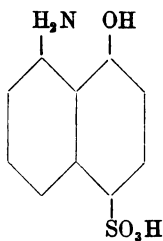
Aminonaphtolsulfosäure S.
